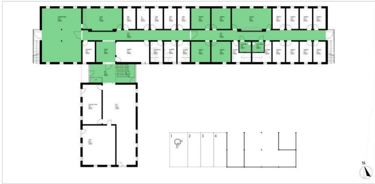
ROLLSTUHLGÄNGIGKEIT E0
