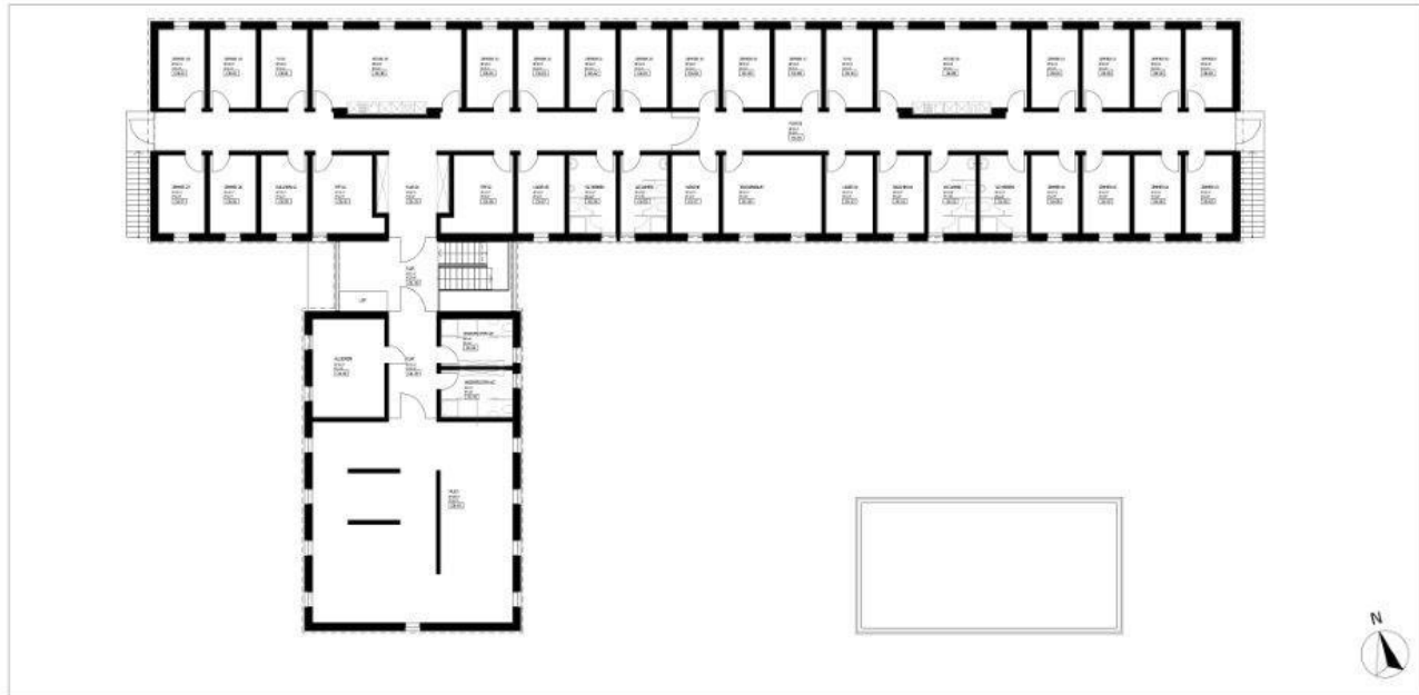
ROLLSTUHLGÄNGIGKEIT O1
